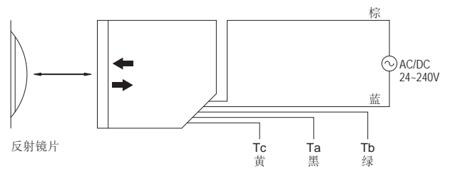
PF系列镜片反射型
