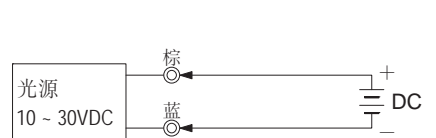
PS, PT系列对照型发射器
